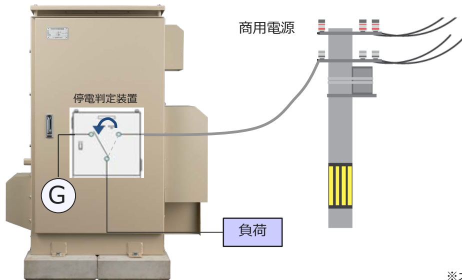
停電時の自動切替モードのイメージ図
